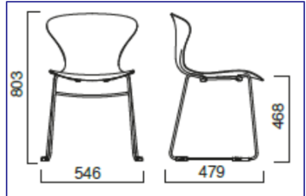
Sled
